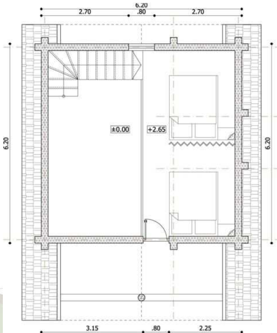
Plan etaj S=19.70 mp
